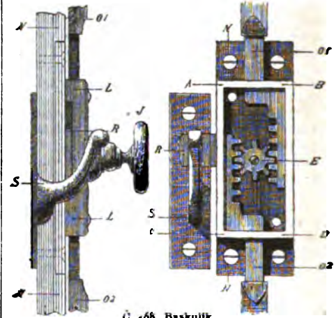
Č. 468. Baskulík.
